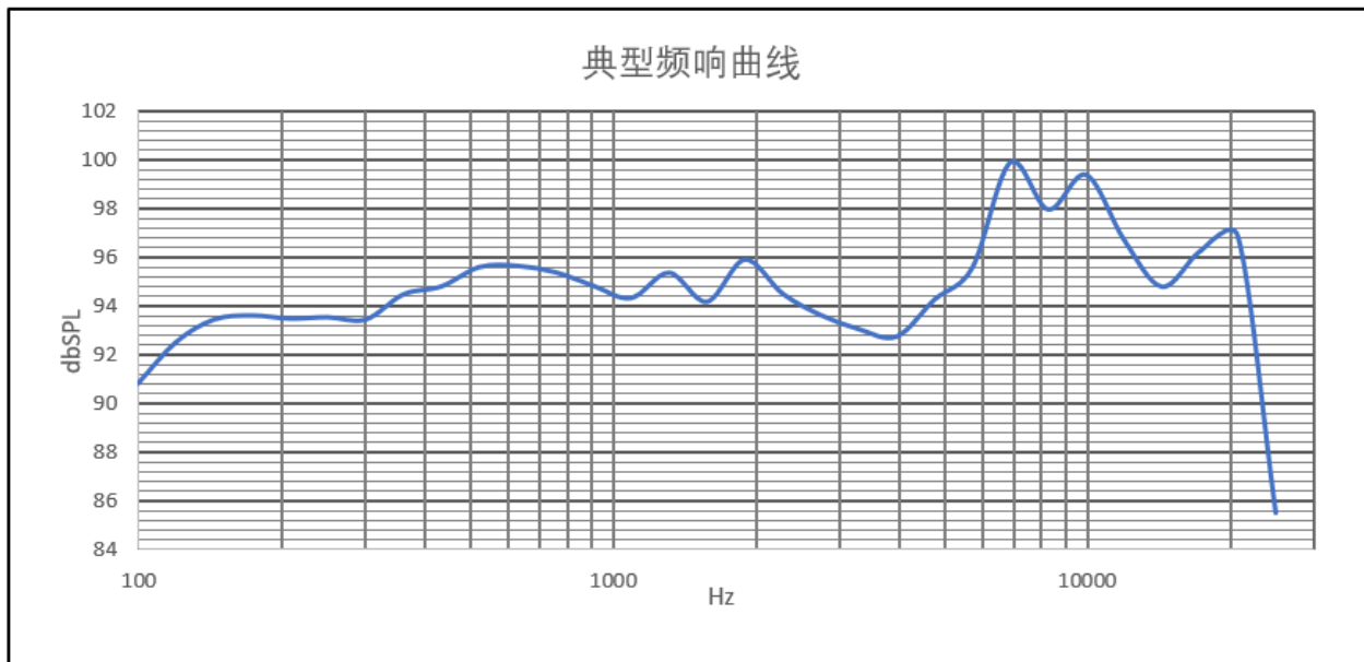
150mm, 1kHz, 94dB SPL 典型频响与失真
